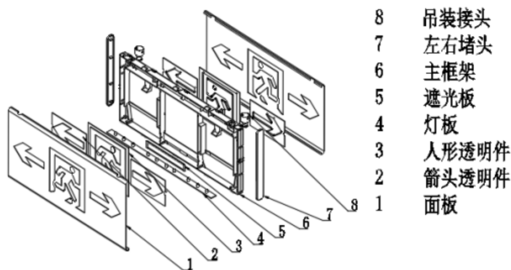
A17 型结构
