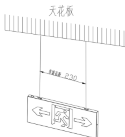
图6 B01B型吊装安装示意图
