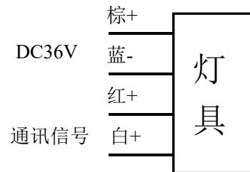
图 5 灯具接线图
