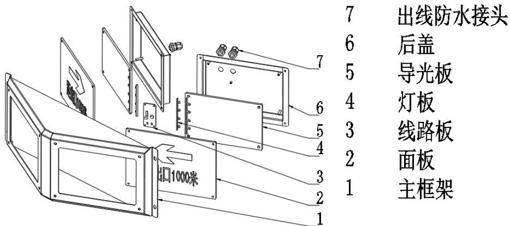
图 2 A25S 系列产品结构图
