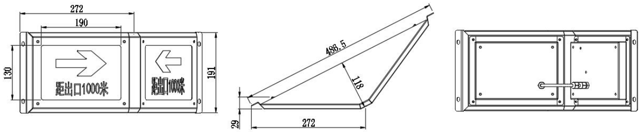
图 1 A25S 系列产品外形图
