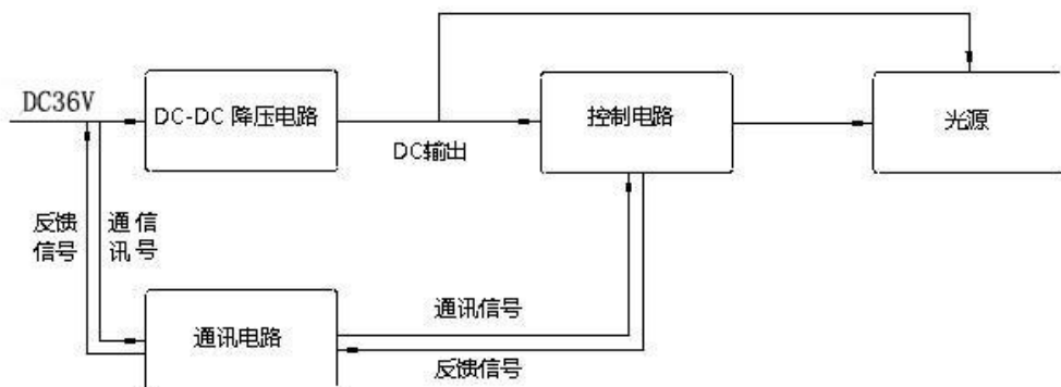
图 3 系统工作原理图
