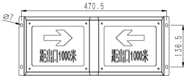
图 4 安装示意图
