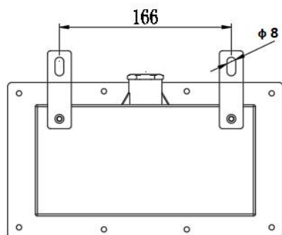
图 4 A01 安装示意图
