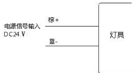
图 5 灯具接线图
