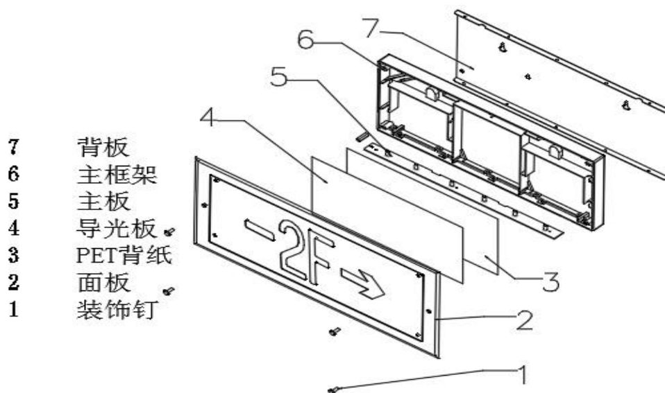
图 2 QA19W 系列产品结构示意图
