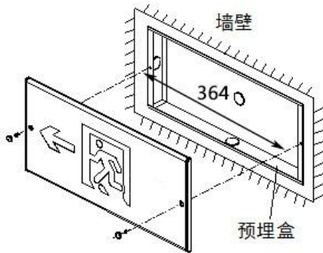
图 4 安装示意图
