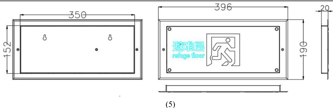
图 1 QA19F 系列外形示意图
