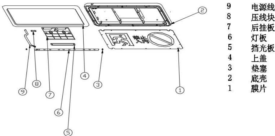
图 2 A901LJ-B 结构图
