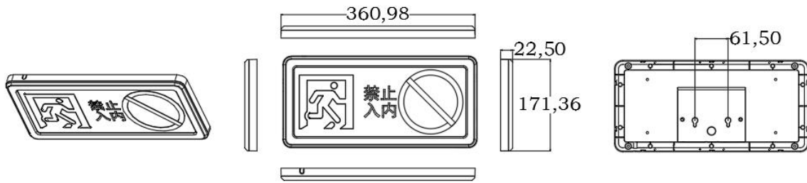
图 1 A901LJ-B 系列产品外形图
