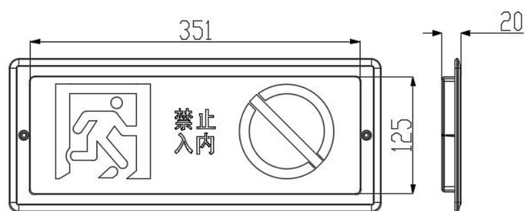
图 1 ZQB01 系列产品外形图
