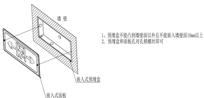
图 4 安装示意图
