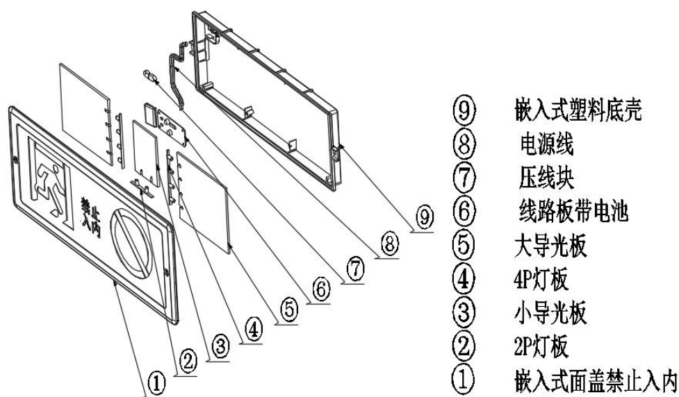
图 2 ZQB01 结构图
