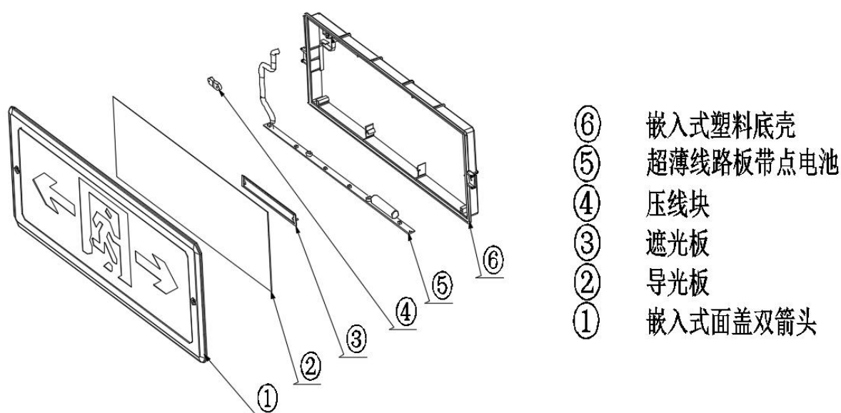
图 2 ZQB01 结构图
