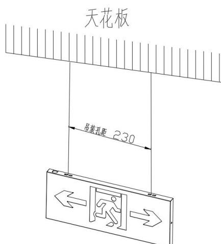
图 5 吊装安装示意图
