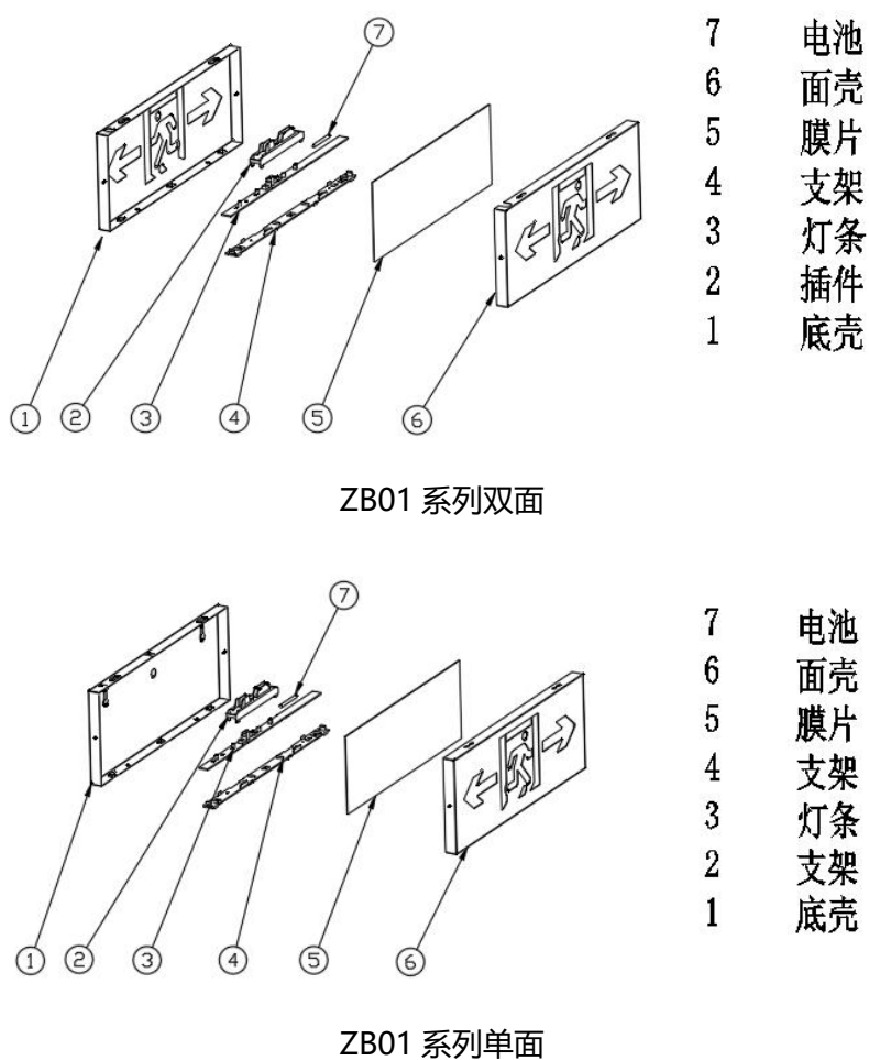
图 2 ZB01 系列结构图
