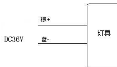
图 6 灯具接线图
