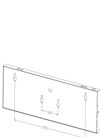
图 4 型单面壁挂安装示意图
