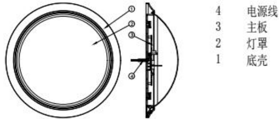
图 2 M07D 结构示意图
