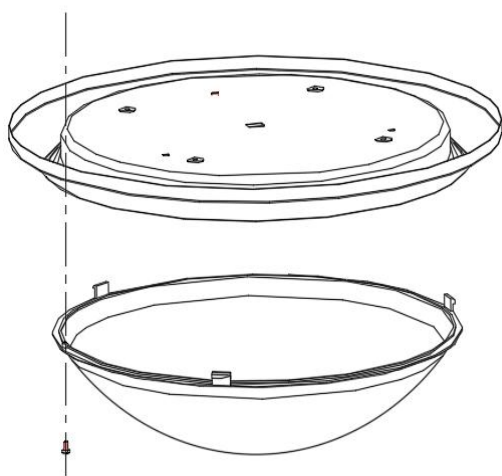
图 6 M07D 外壳安装示意图
