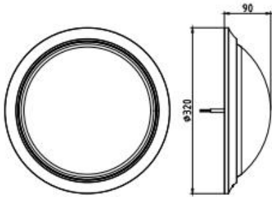
图 1 M07D 外形示意图
