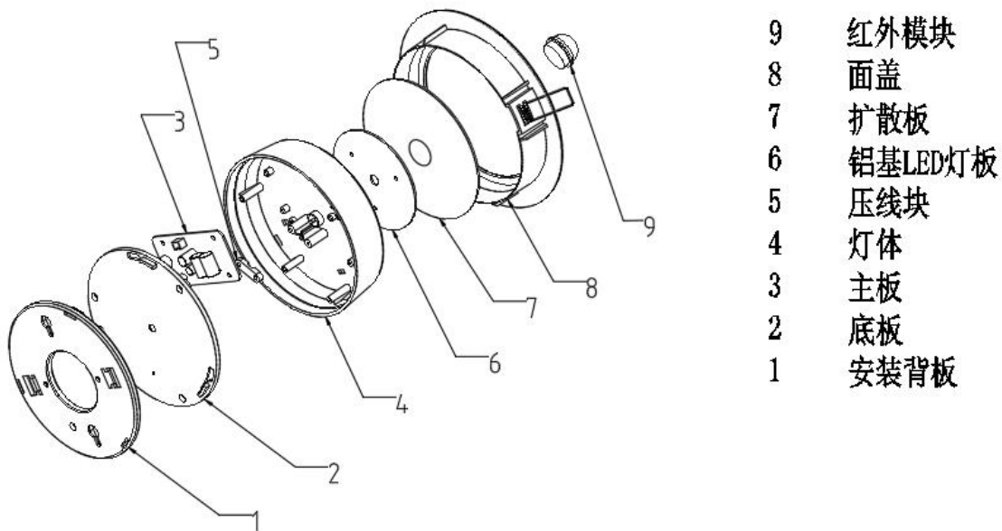
图 2 结构示意图
