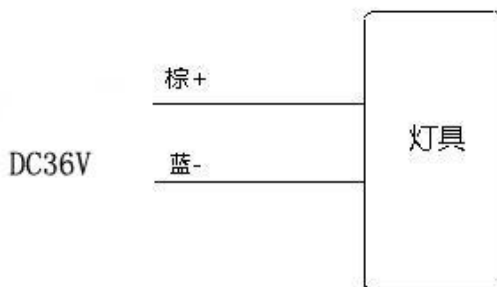
图 4 QS08 安装示意图
