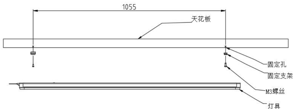
图 4 T8-12H 安装示意图
