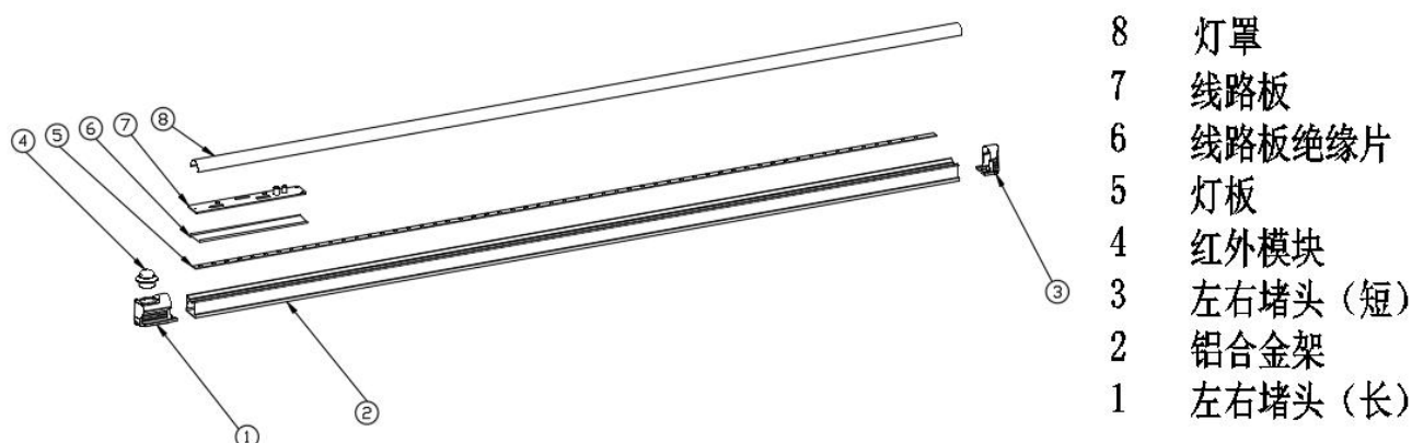
图 2 T8-12H 型结构示意图
