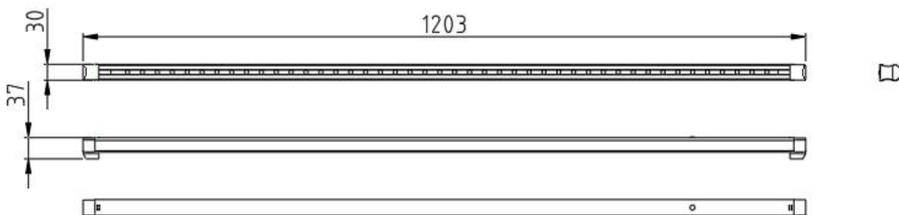
图 1 T8-18 系列外形示意图
