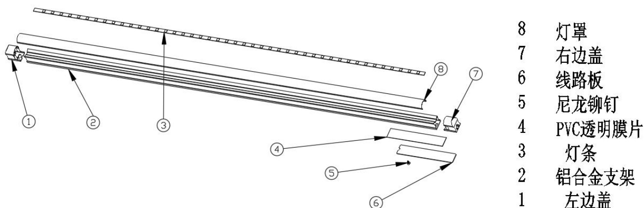
图 2 T8-18 系列结构示意图
