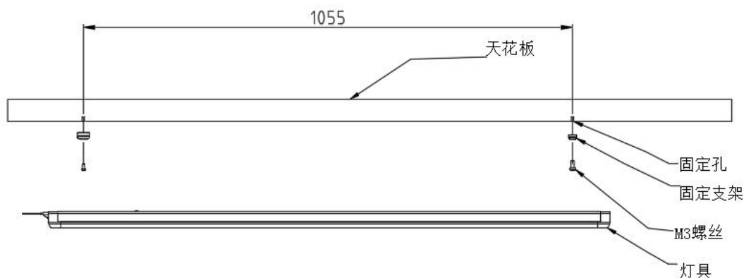
图 4 T8-18 安装示意图
