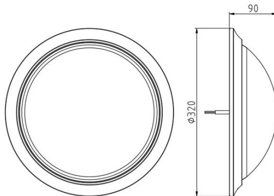
图 1 ZM07-Y5 系列外形示意图
