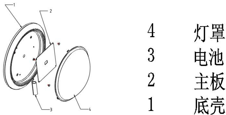
图 2 ZM07-Y5 系列产品结构示意图
