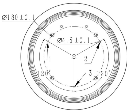
图 4 ZM07-Y5 系列底壳孔位图
