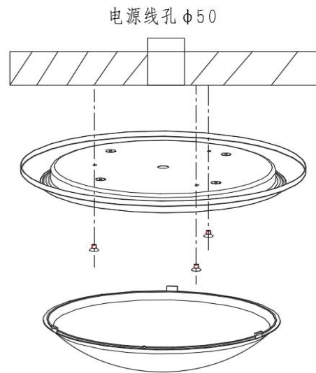
图 5 ZM07-Y5 系列底壳安装示意图
