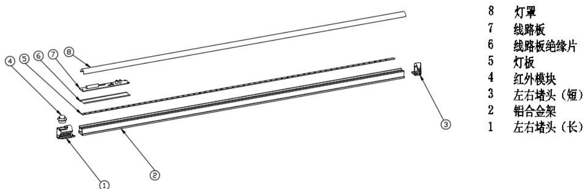
图 2 ZT8-18H 型结构示意图
