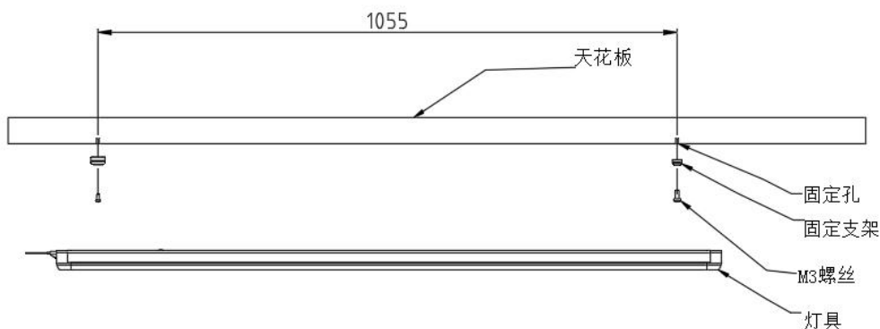
图 4 ZT8-18H 安装示意图
